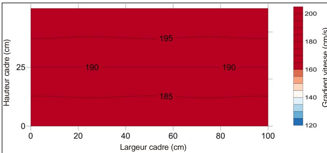
Figure 6 : Mesures à vitesse rapide.
