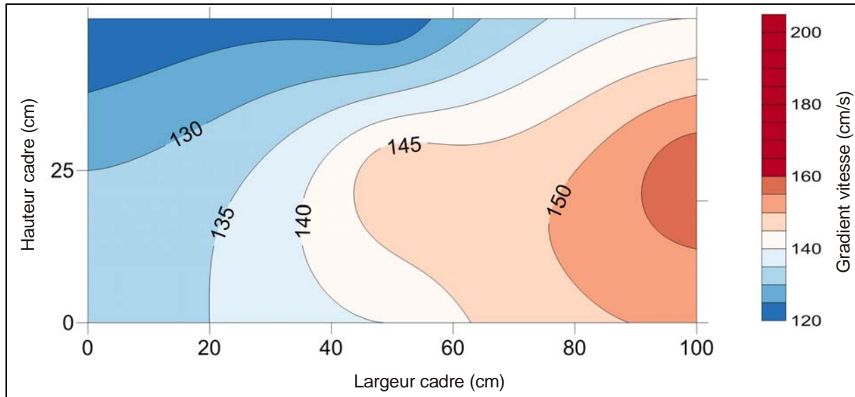
Figure 3 : Mesures à vitesse lente.
