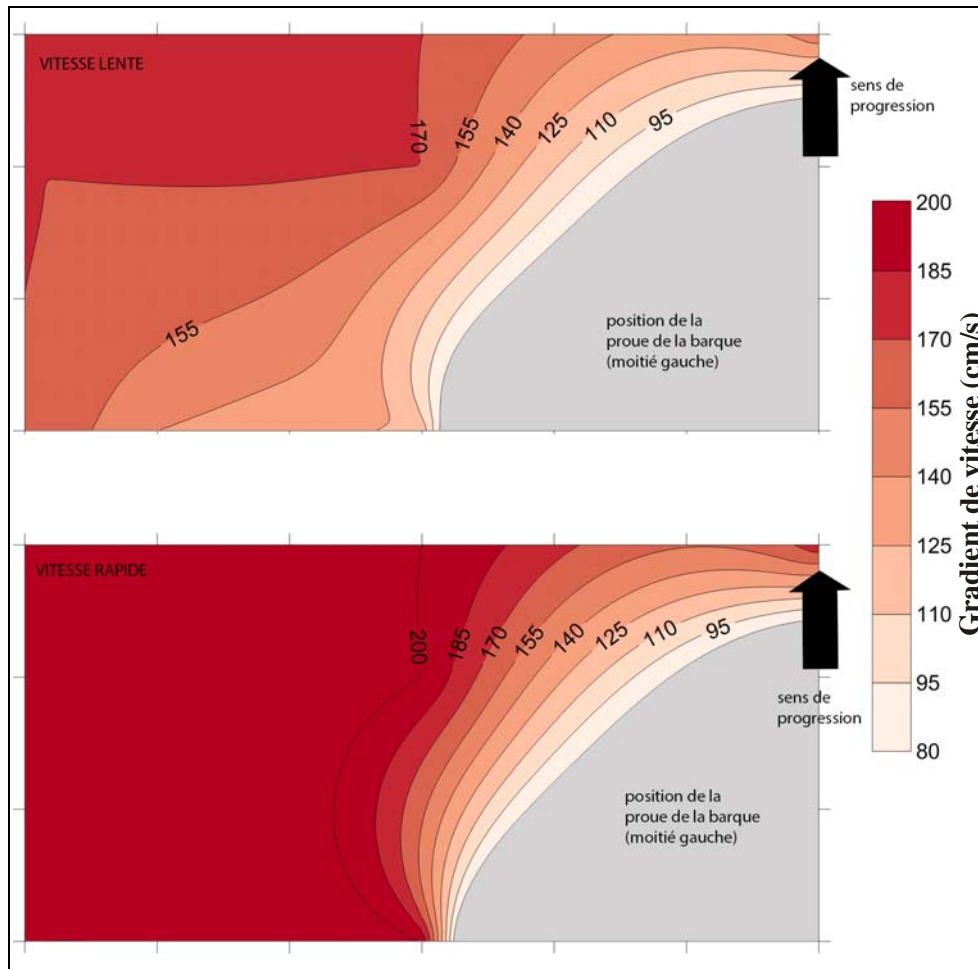
Figure 2 : Ecoulements à la proue du bateau.
