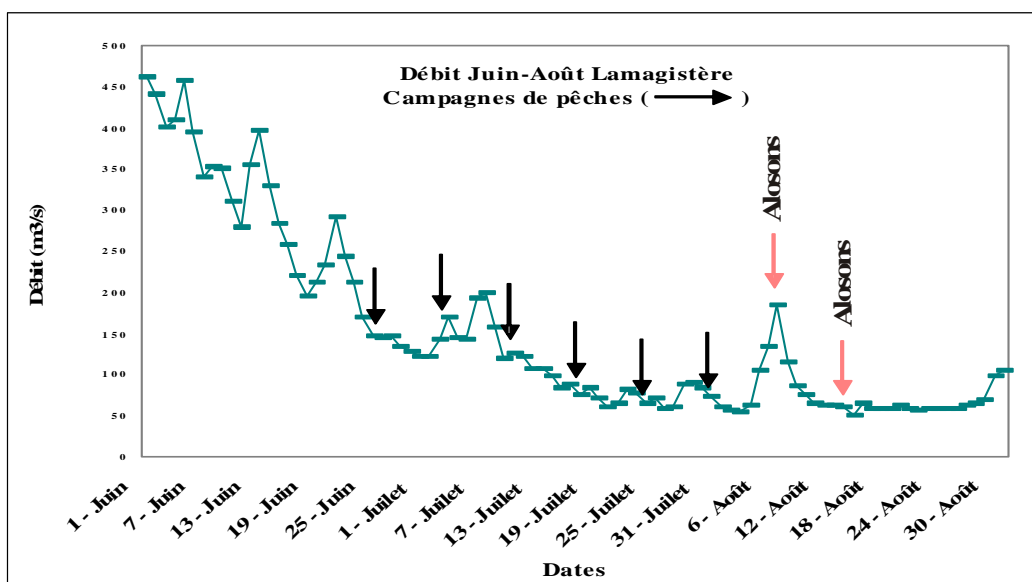
Figure 7 : Evolution des débits de la Garonne à Lamagistère de Juin à Août 2012
