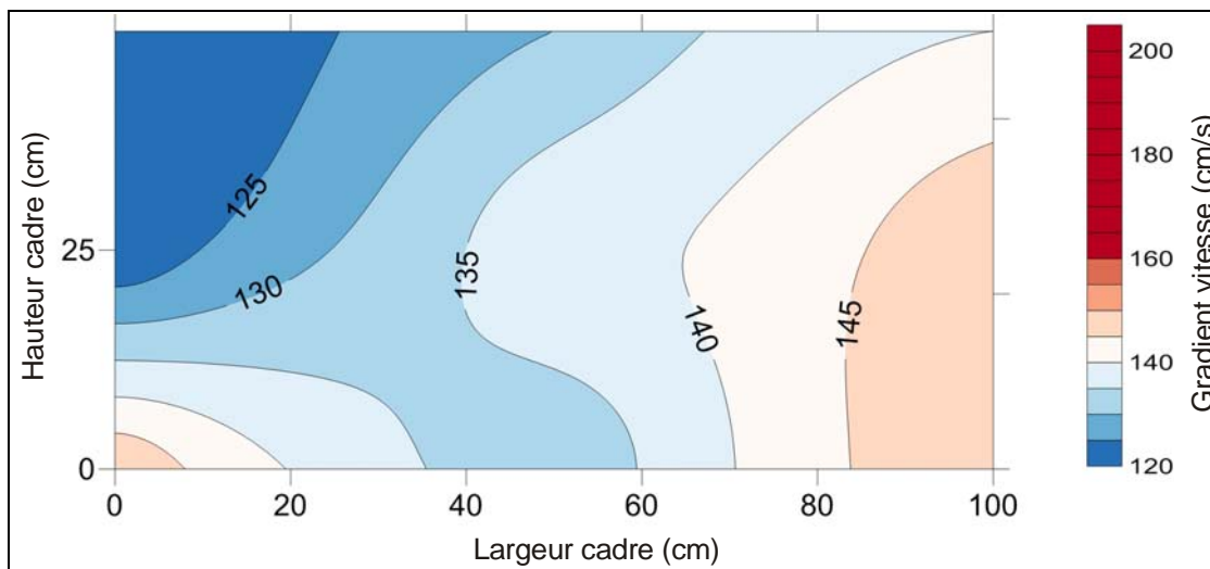
Figure 5 : Mesures à vitesse lente.
