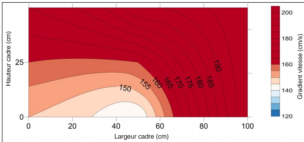
Figure 4 : Mesures à vitesse rapide.
