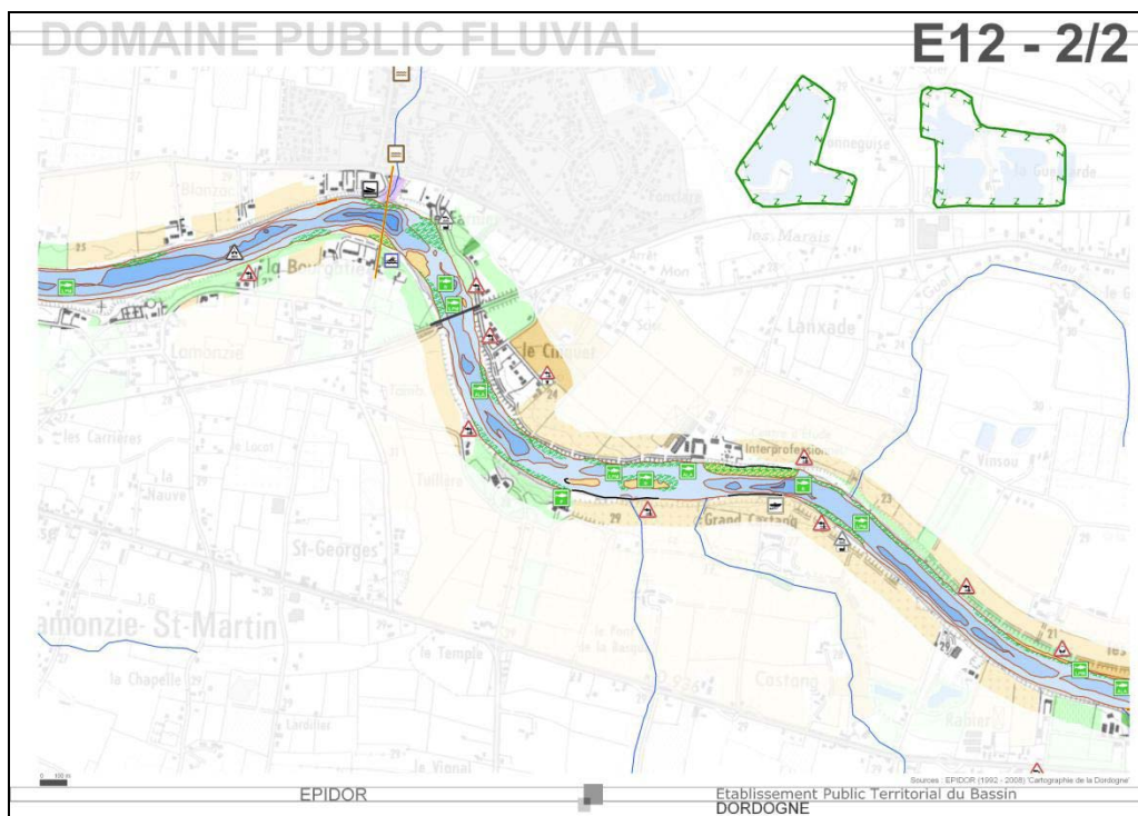
Carte 5 : Bathymétrie du site de pêche (source EPIDOR).
