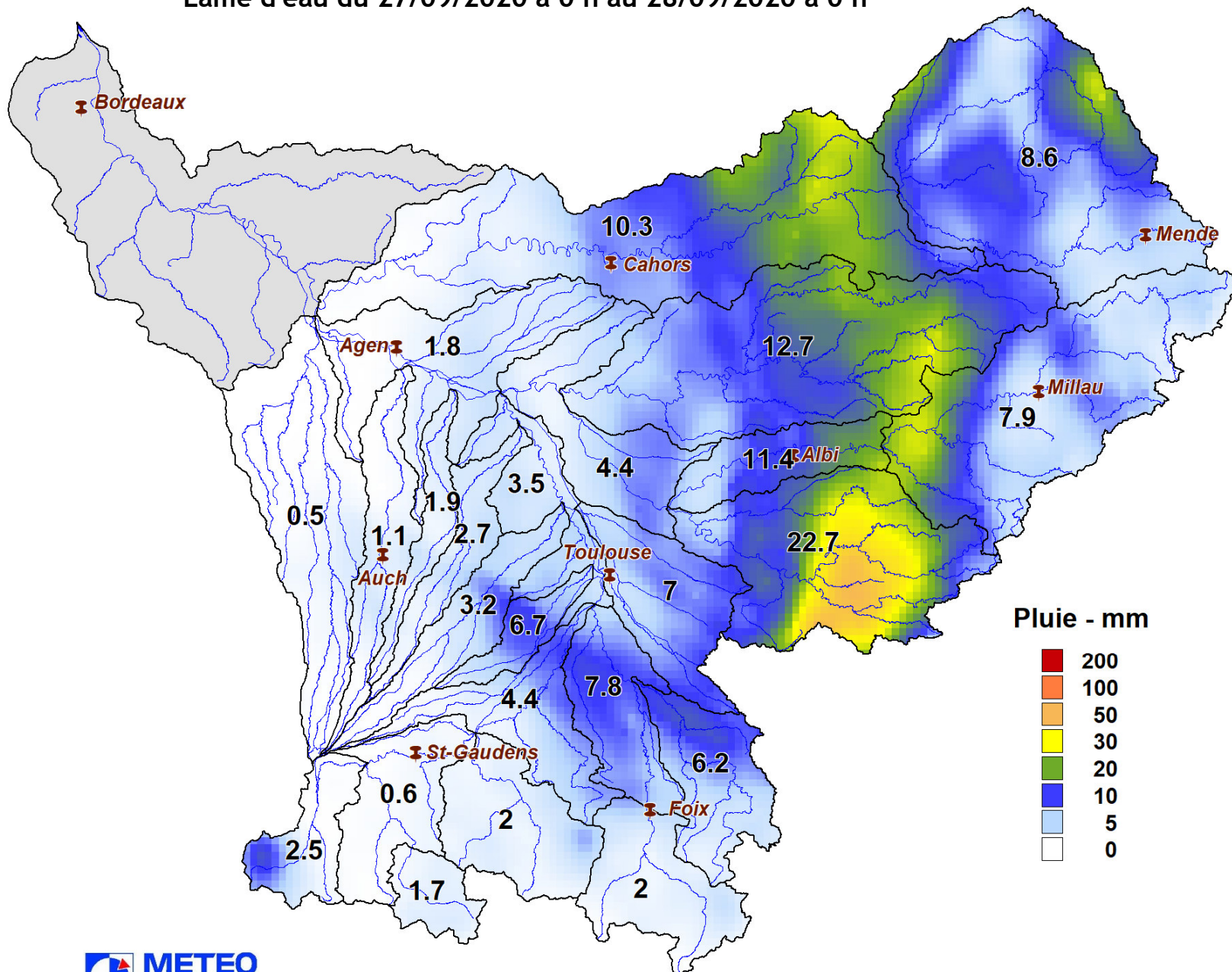
Lame d'eau du 27/09/2020 à 0 h au 28/09/2020 à 0 h
