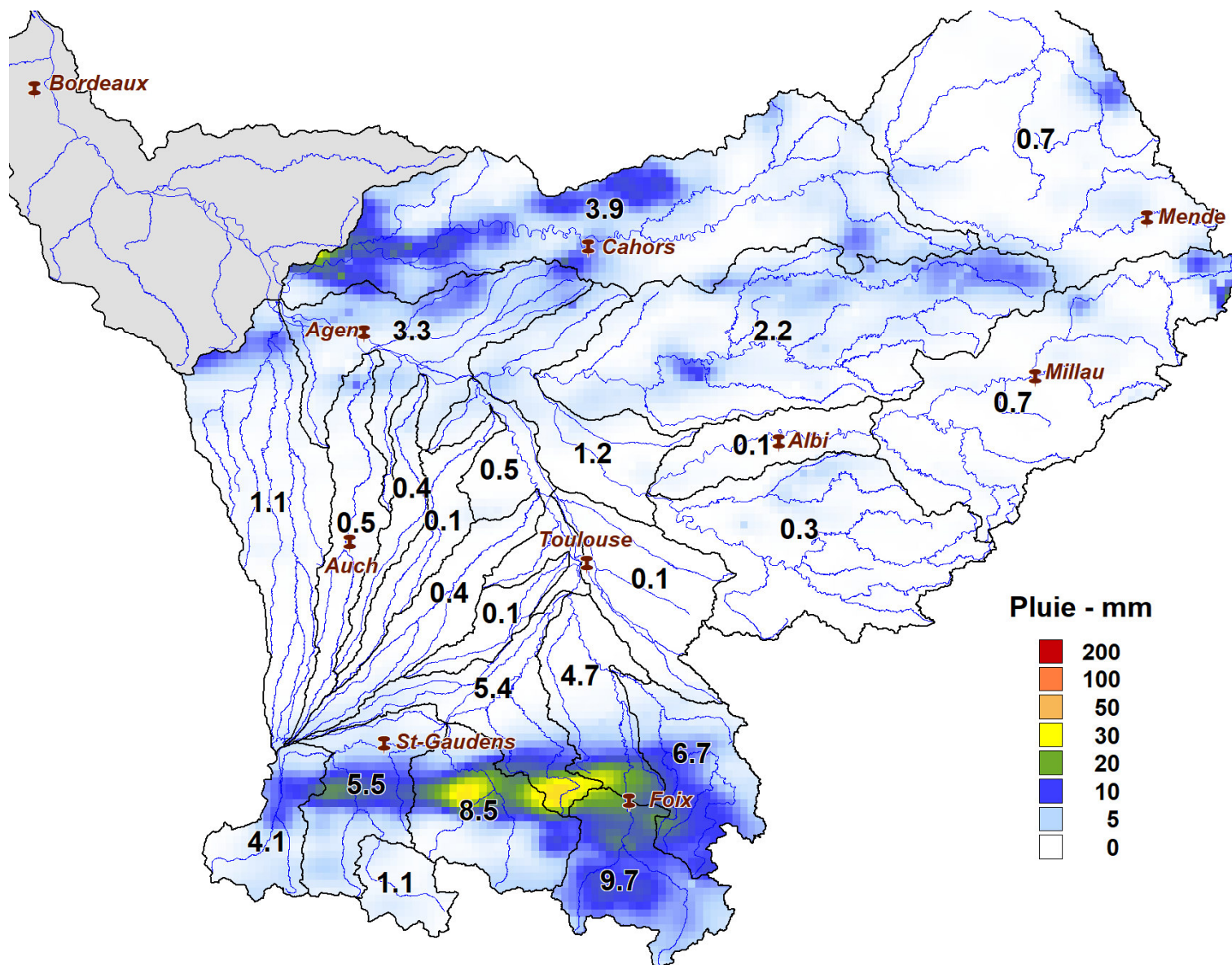
Lame d'eau du 20/09/2020 à 0 h au 21/09/2020 à 0 h
