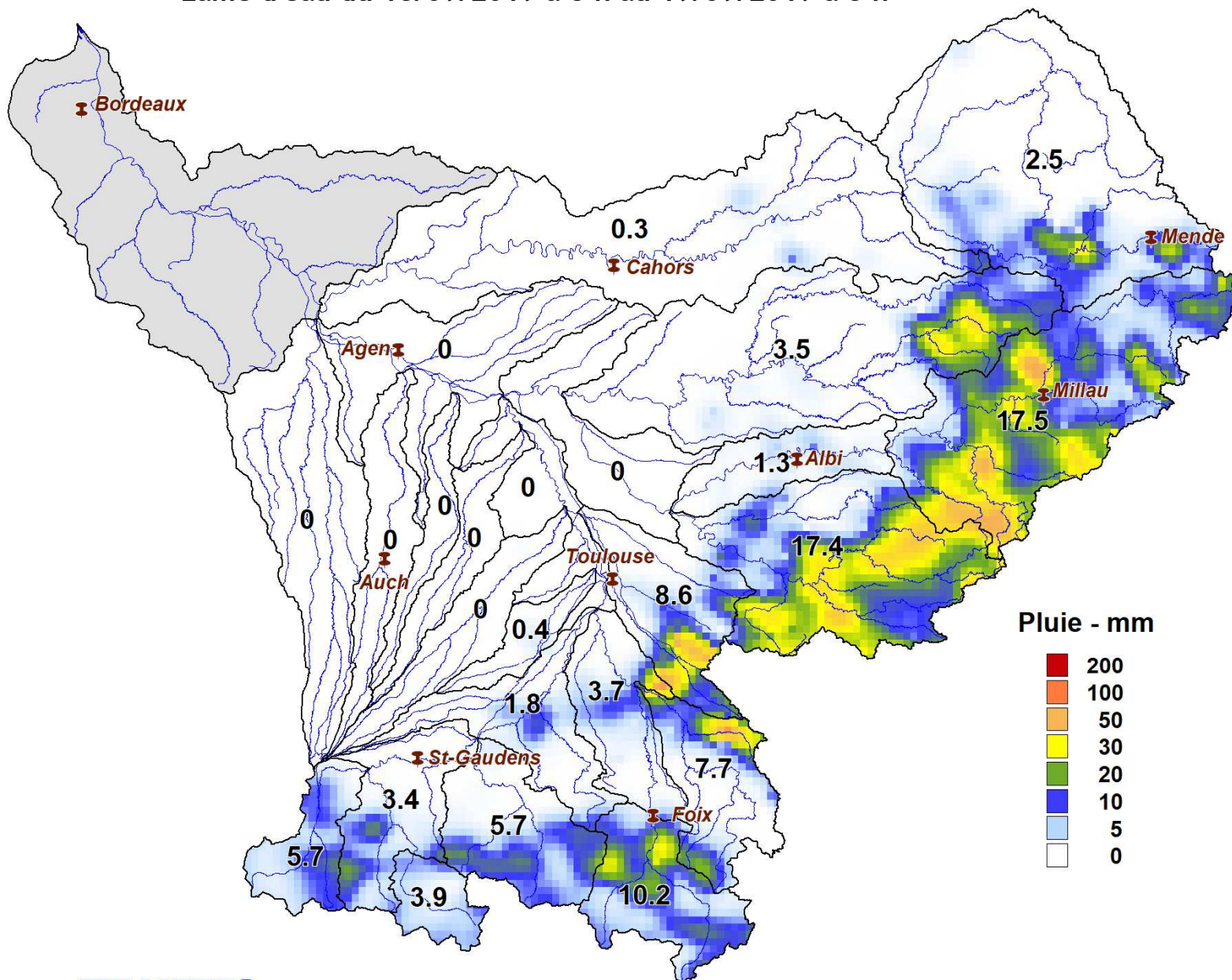
Lame d'eau du 18/09/2019 à 8 h au 19/09/2019 à 8 h
