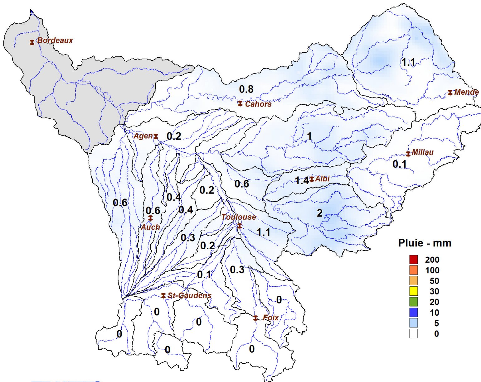
Lame d'eau du 15/07/2020 à 0 h au 16/07/2020 à 0 h
