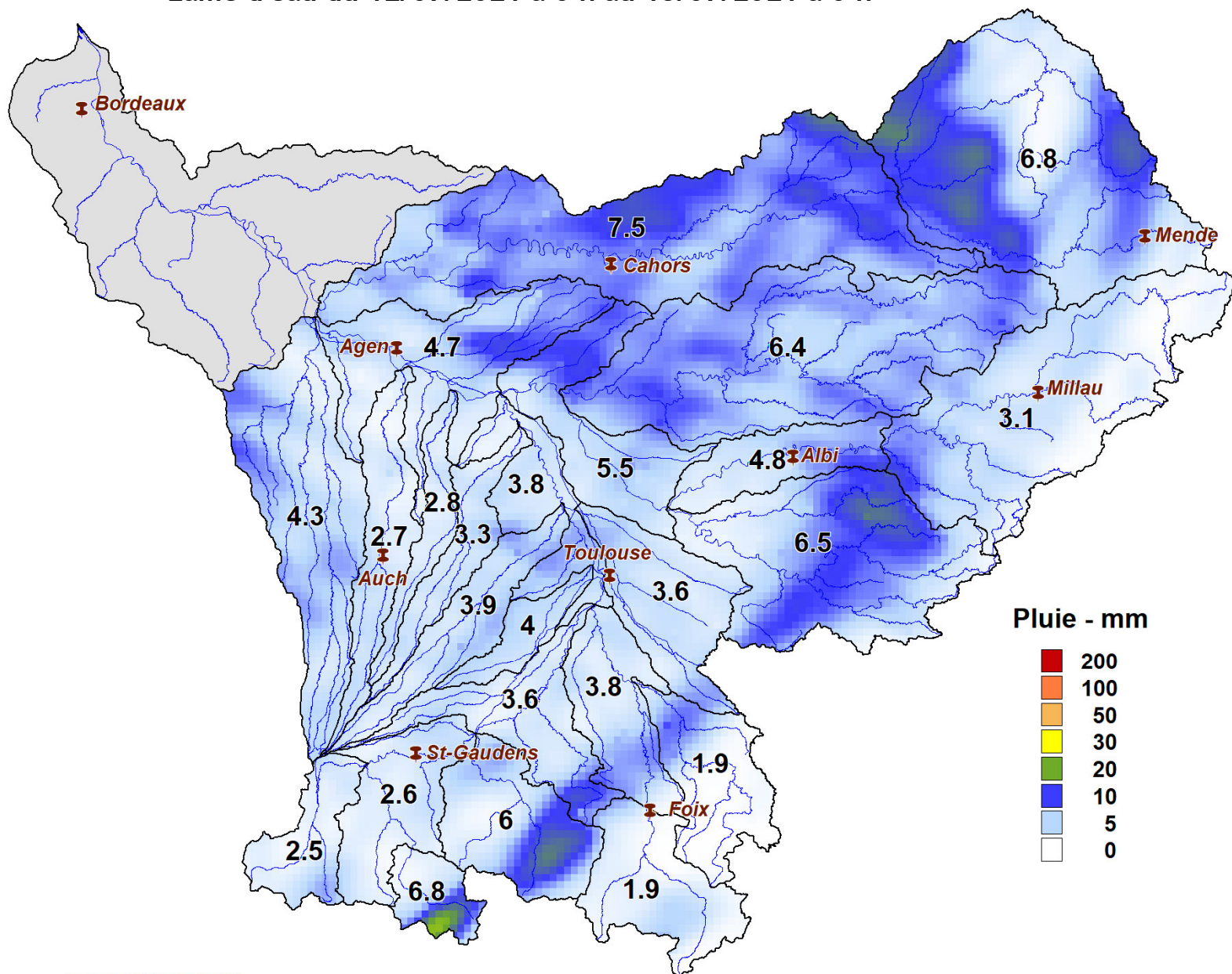
Lame d'eau du 12/07/2021 à 0 h au 13/07/2021 à 0 h
